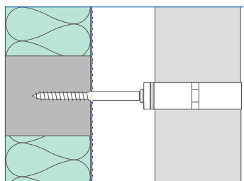
Rohrschellen mit Holzgewinde
