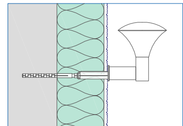
Lampen
