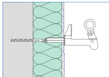
Klappladenarretierung
