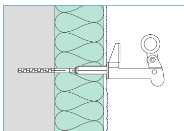
Klappladenarretierung
