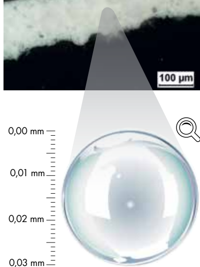
Einzelne Microhohlglasskugel, ca. 1.100-fach vergrößert
